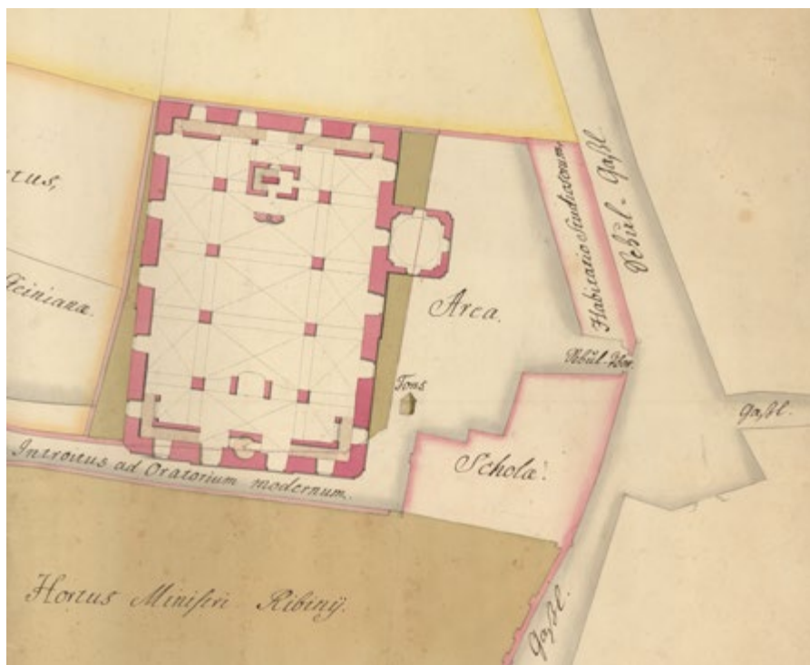
Obr. 1: Situačný plán z výkresu projektu Nemeckého evanjelického kostola, zachytávajúci aj pôdorysnú stopu komplexu budov evanjelických škôl pred výstavbou nového objektu. Autor neuvedený. Archív mesta Bratislavy, Zbierka máp a plánov, inv. č. 1369 (výrez).
